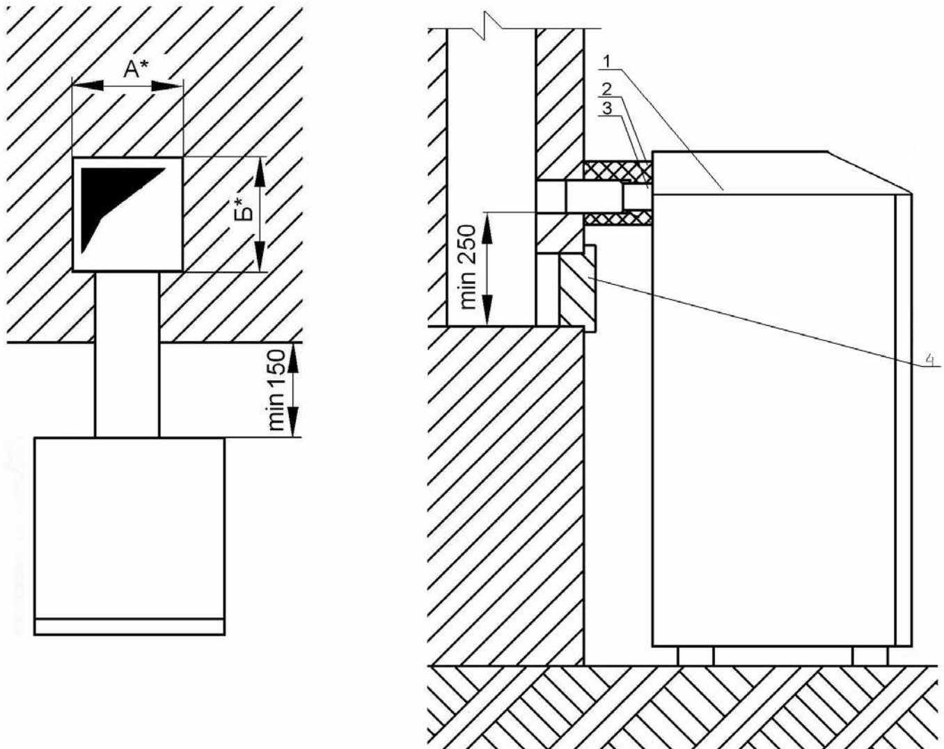
Соединение патрубка для отвода продуктов сгорание с дымовым каналом
